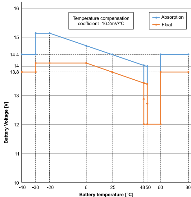
Temperaturkompenserat laddningsdiagram
