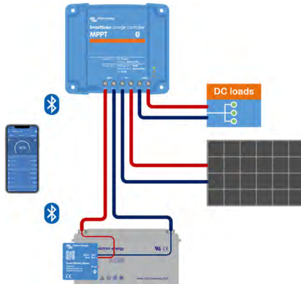
Exempel på ett VE.Smart Network med en Smart Battery Sense och en solcellsladdare.
